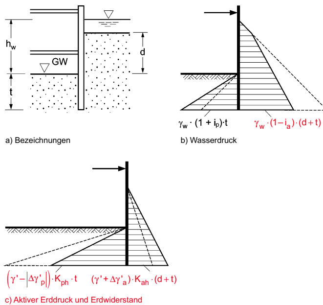
Bild EB 63-2. Aktiver Erddruck, Wasserdruck und Erdwiderstand bei einer umströmten Baugrubenwand im Wasser (vereinfachte Darstellung)
